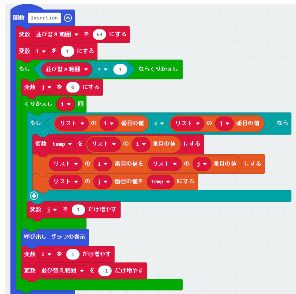
図6 プログラム例（挿入ソートの一部）
