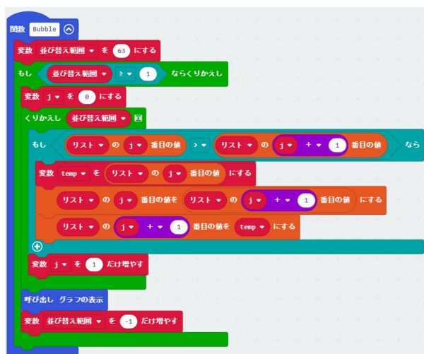
図5 プログラム例（バブルソートの一部）
