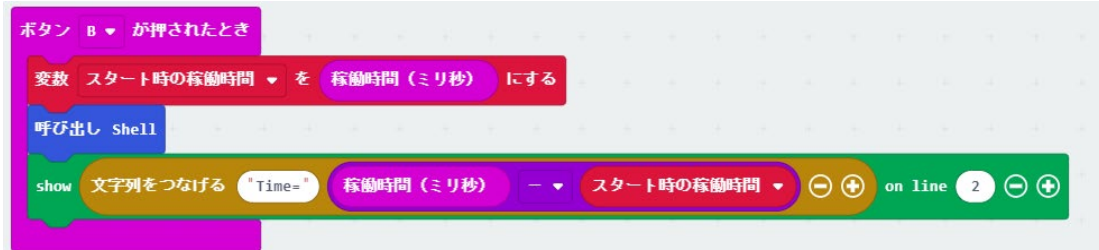
図4 内部タイマーを使ったソートの稼働時間の計算とその表示プログラム
